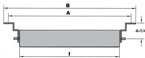
RODILLO DE RETORNO
