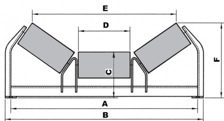
TRIPLE RODILLO DE CARGA A 20°
