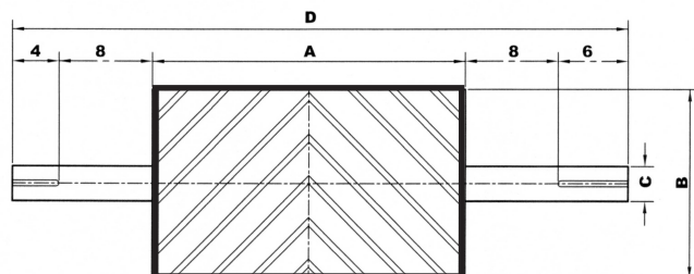
POLEA MOTRIZ
