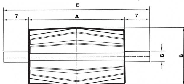
POLEA DE COLA
